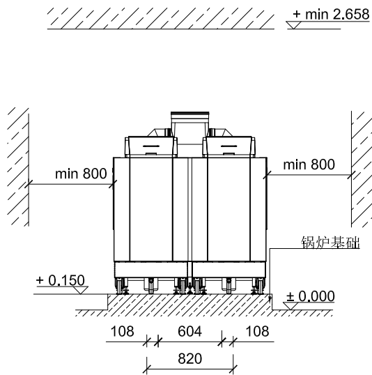
主视图
