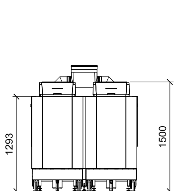
主视图
