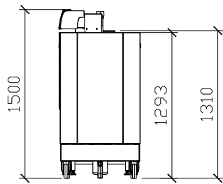
主视图
