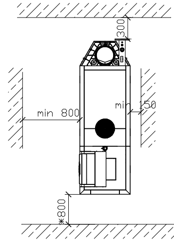
俯视图
