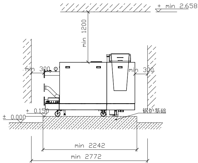
侧视图
