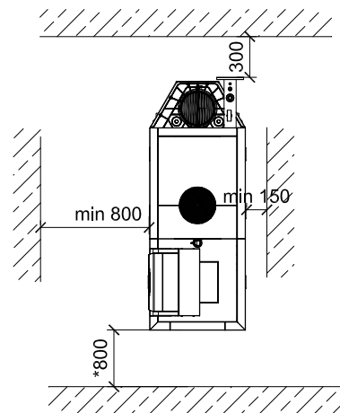
俯视图
