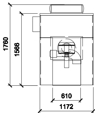
主视图
